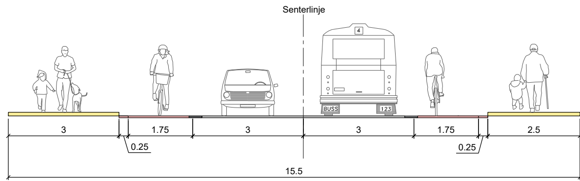
Sykkelfelt med fortau
