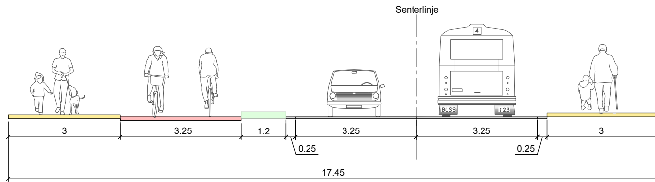
Gang-/sykkelveg med fortau
