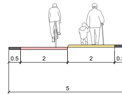
Envegsregulert sykkelveg med fortau i tunnel
