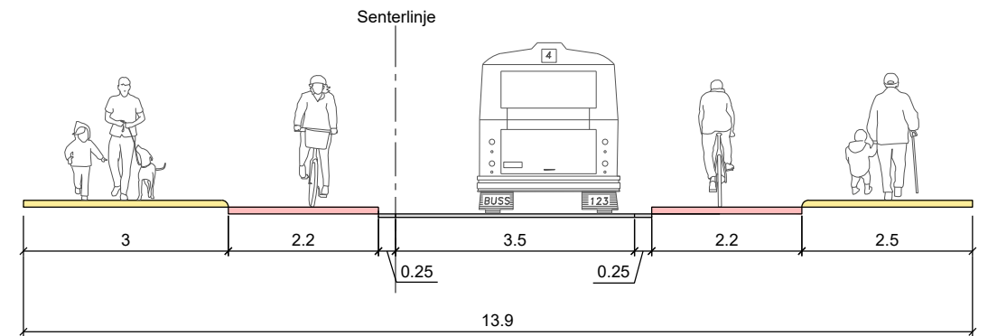
Envegsregulert sykkelveg med fortau v/små kjørebane
