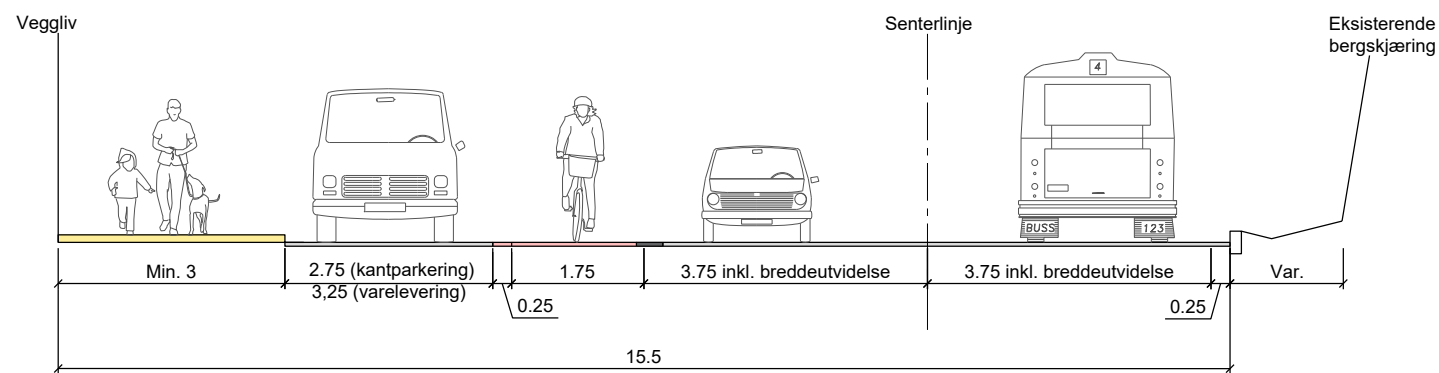
Sykkelfelt med varelevering/kantparkering
